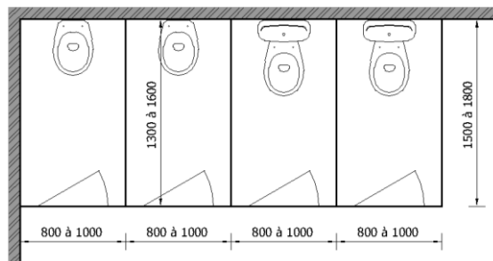
CABINES TOILETTES AVEC PORTES OUVRANT VERS L'INTÉRIEUR
