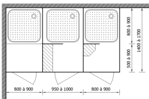
CABINES DOUCHES AVEC LES PORTES OUVRANT VERS L'EXTÉRIEUR
