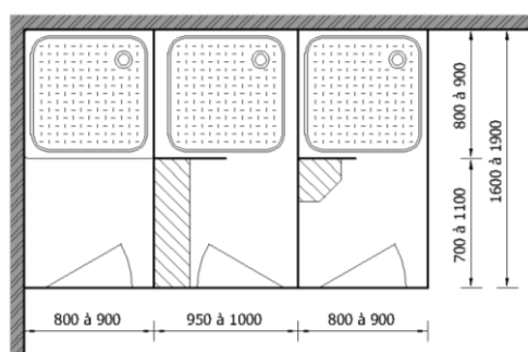
CABINES DOUCHES AVEC PORTES OUVRANT VERS L'INTÉRIEUR
