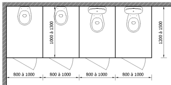
CABINES TOILETTES AVEC LES PORTES OUVRANT VERS L'EXTÉRIEUR
